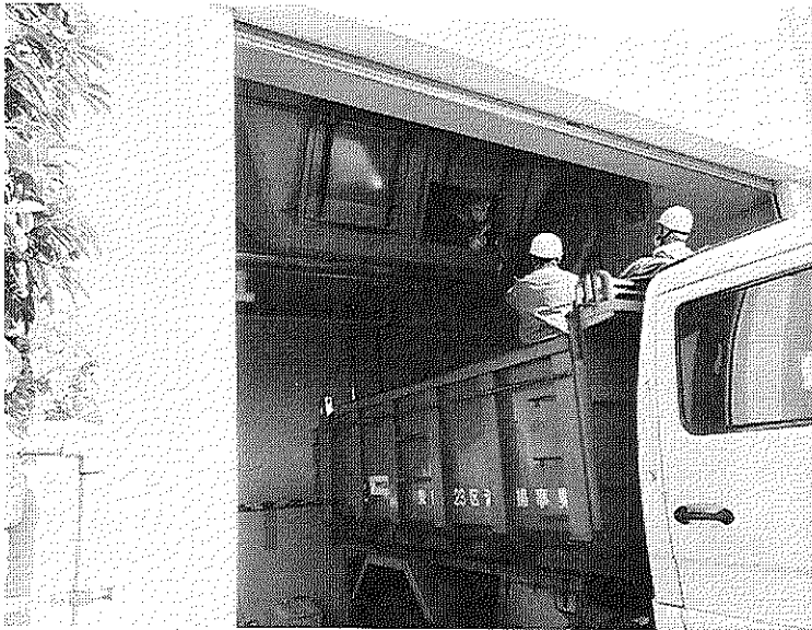
▲常に危険が伴うホッパー作業は反転コンテナへと要求
